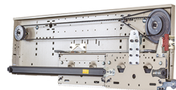
درب کابین تلسکوپی نیمه اتوماتیک دو لته ۴ سانتی
