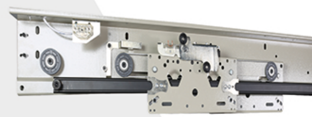
درب طبقه تلسکوپی تمام اتوماتیک ۲ لته ۴ سانتی طرح فرماتوری
